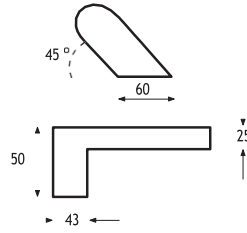
Manillon desplazado 45° 45° simple outer pull handle
